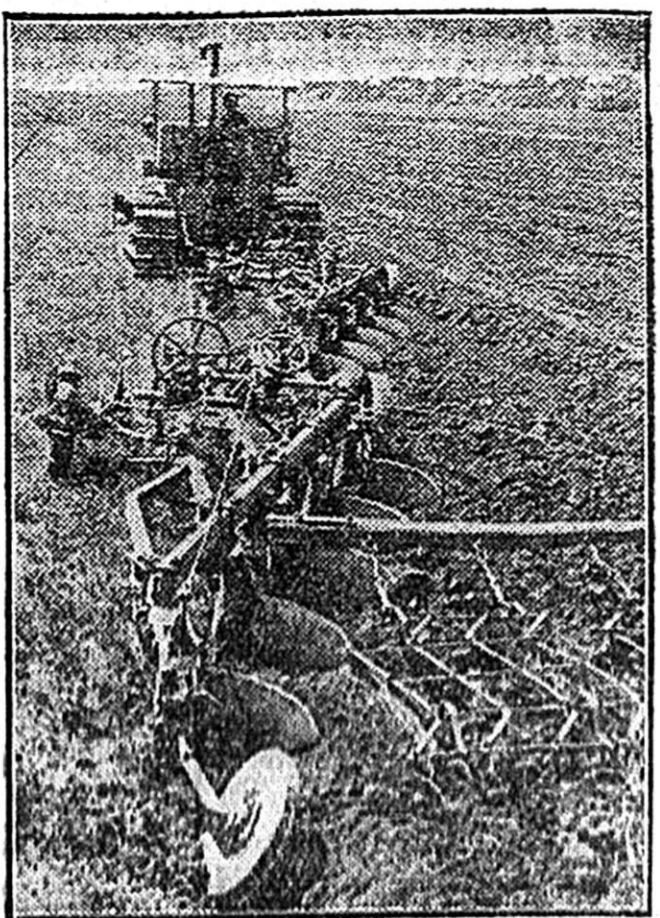
Itt az őszi szántás! Az „Sz-80-as” traktor két testű ökhántolós ekét húz s a szántással együtt a boronálás munkáját is elvégzi.
